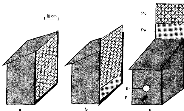
Figure 2. Nichoirs de type I (à parois amovibles). E entrée; P perchoir; Pc paroi amovible en contreplaqué; Pv paroi amovible en verre.
